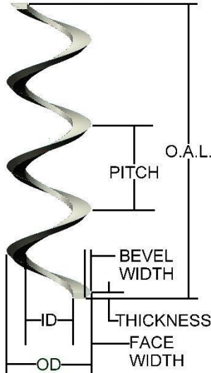
Beveled Edge Auger
